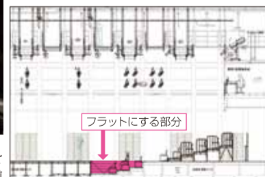
(舞台断面図)向かって左がステージ。今回は前方客席をフラットにする
